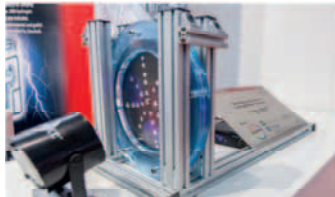
Abbildung 2: Teststand auf dem Stand der Firma Eisenhuth zur Hannover Messe zum Forschungsprojekt RADAR
