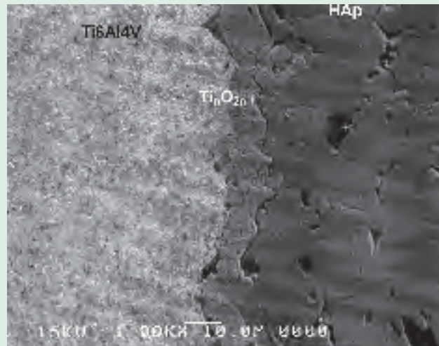
Bild 5: Rasterelektronenmikroskopische Aufnahme eines Querschnitts eines biokeramischen Schichtsystems Links: bioinertes Ti6Al4V-Implantat, Mitte: bioinerte Haftvermittlerschicht aus TiO_{2n-1} Rechts: biokonduktive HAp-Schicht (HEIMANN 1999)
