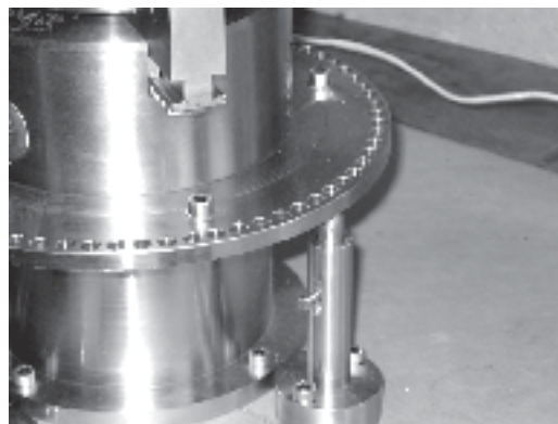
Bild 8: Detail der Dreh- und Positioniereinrichtung
