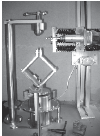
Bild 7: Bohr- und Fräsvorrichtung
