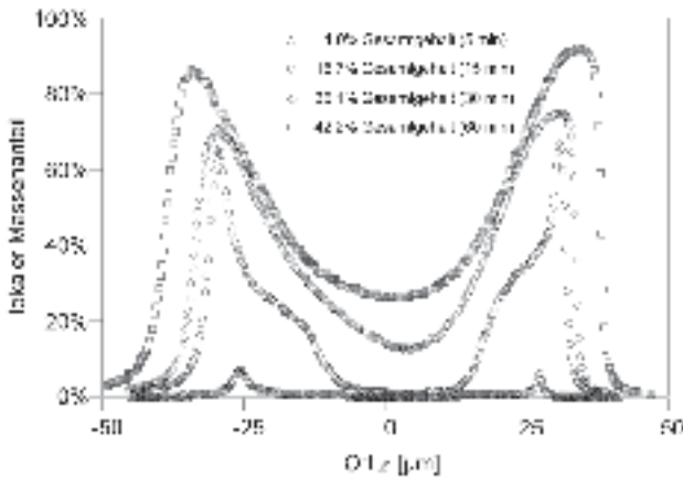
Bild 6: (a) Schnittbilder durch vier fluoridierte Polymermembranen, hergestellt am Institut für Technische Chemie, mit (von links nach rechts) zunehmendem Gehalt an Pfp-Copolymer (Polystyrol). (b) Die zugehörigen Konzentrations-Orts-Profile. Der Pfp-Copolymergehalt nimmt mit zunehmender Reaktionszeit zunächst an den Membranoberflächen, später auch in der Membranmitte zu.
