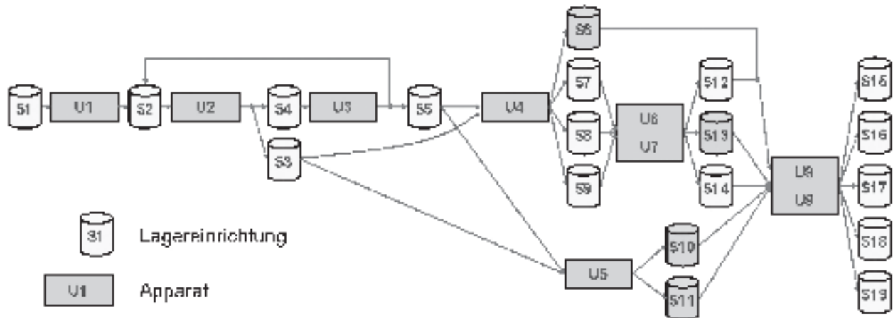
Bild 1: Verfahrenstechnische Mehrzweckanlage
