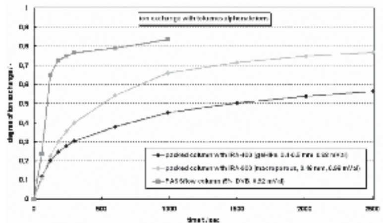
Bild 4: Vergleich der Ionenaustauschgeschwindigkeit von monolithischen Composit-Reaktoren mit handelsüblichen Ionenaustauschern. Austausch von Chlorid gegen Toluolsulfonat
