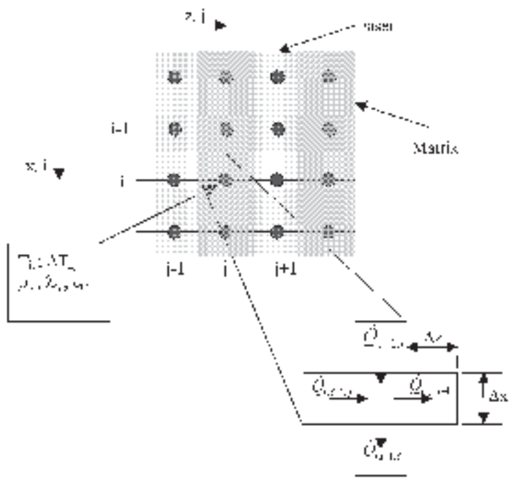
Bild 2: Gitternetz zur Bestimmung des zweidimensionalen Wärmestromes
