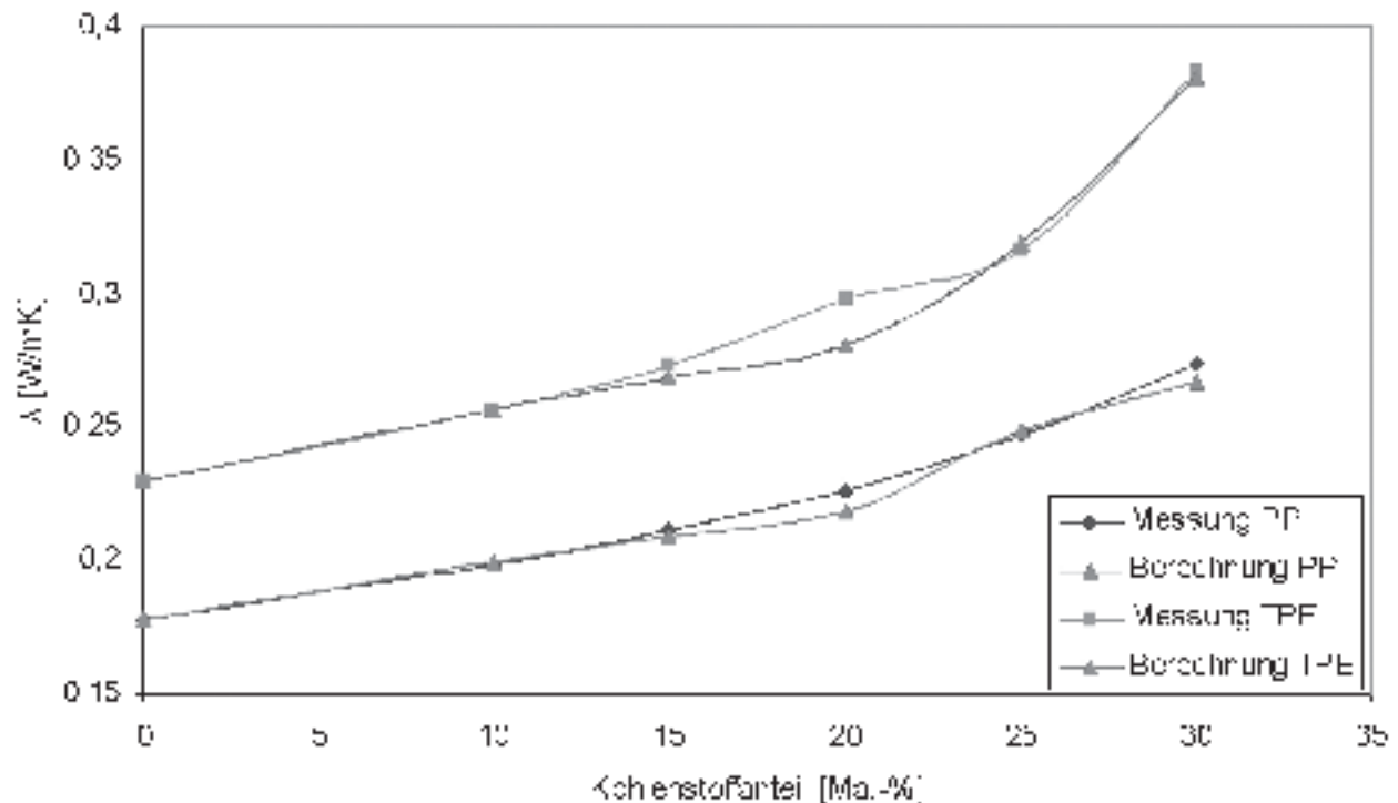
Bild 5: Vergleich der berechneten und experimentell ermittelten Wärmeleitfähigkeit
