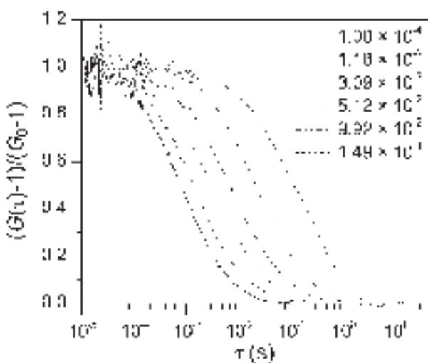
Bild 8: Typische Autokorrelationskurven aus einer FCS-Messung (durchgeführt von R. Liu, Institut für Physikalische Chemie) an fluoreszenzmarkierten Polystyrolmolekülen in Polystyrollösungen unterschiedlicher Konzentrationen (angegeben in g/mL).
