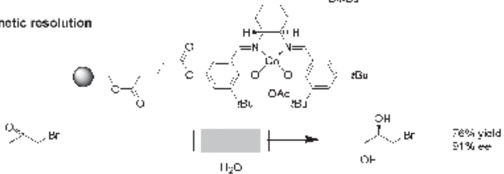
Schema 2: Umsetzungen mit Übergangsmetallkatalysatoren
